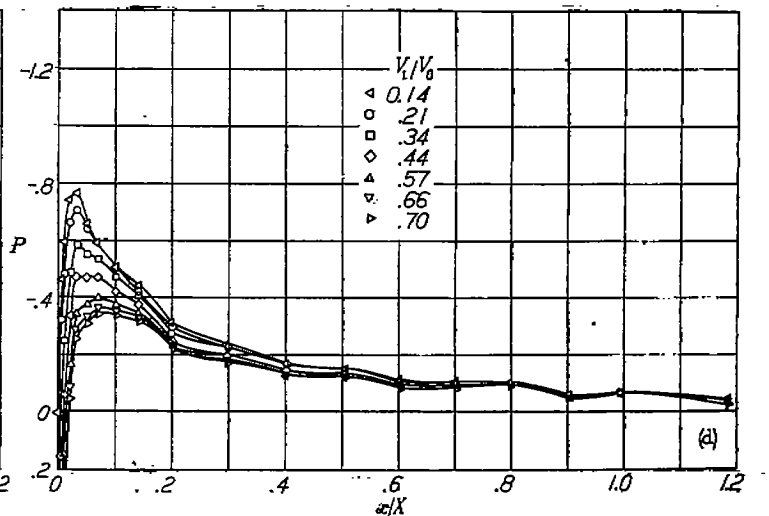
(a) NACA 1-60-160 nose inlet; M_0=0.30 . (b) Elliptical; M_0=0.30 . (c) K=0.5 ; M_0=0.40 . (d) K=1.5 ; M_0=0.40 .
