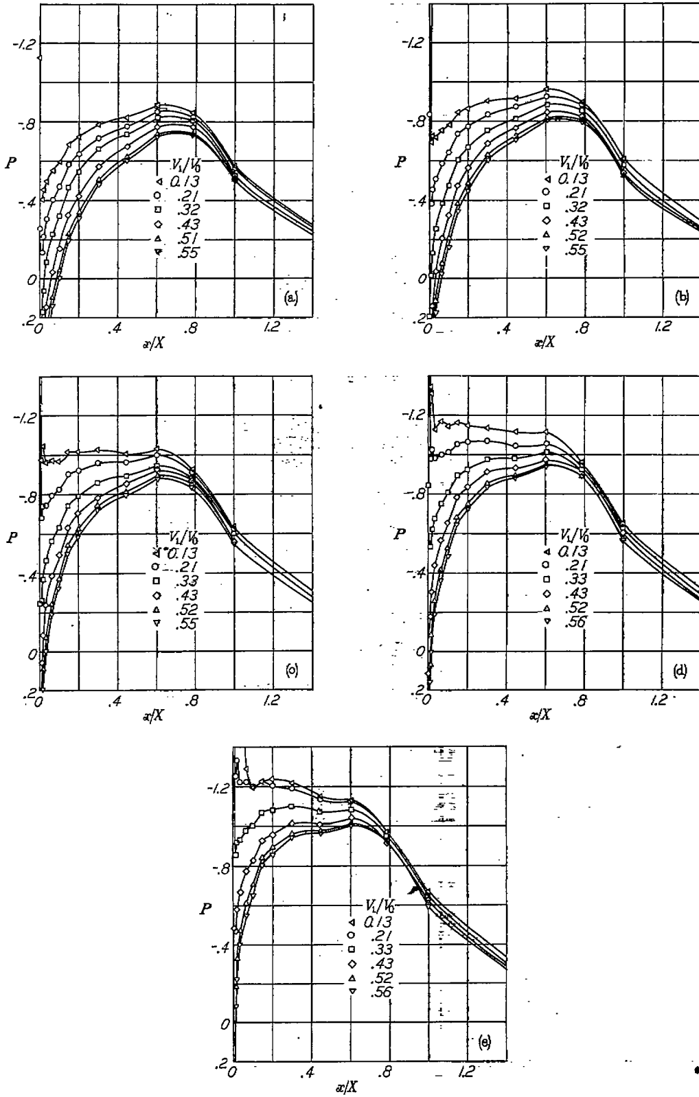
(a) \alpha = -0.1^\circ . (b) \alpha = 1.8^\circ . (c) \alpha = 3.8^\circ . (d) \alpha = 5.8^\circ . (e) \alpha = 7.8^\circ .
