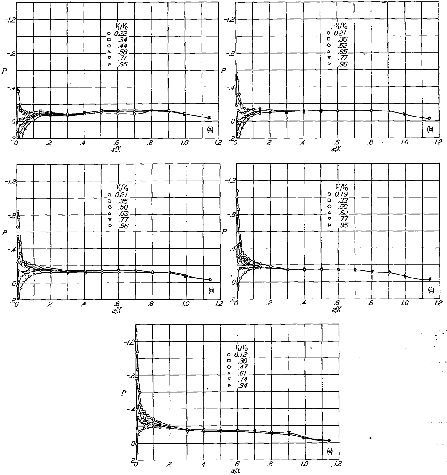
(a) \alpha = -0.2^\circ . (b) \alpha = 1.9^\circ . (c) \alpha = 3.9^\circ . (d) \alpha = 5.8^\circ . (e) \alpha = 7.3^\circ .
